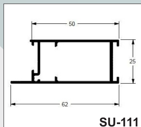
Montante
