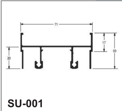
Marco superior
