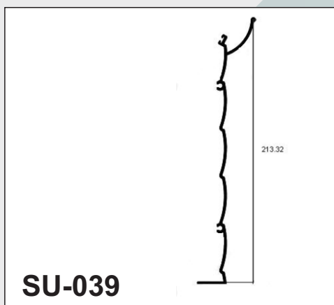
Trilho superior
