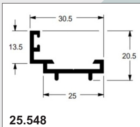
Batente
