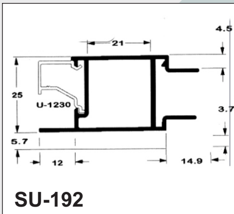
Montante central
