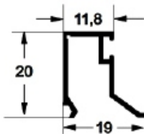
L 1027 - Baguetinho
