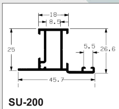
Montante
