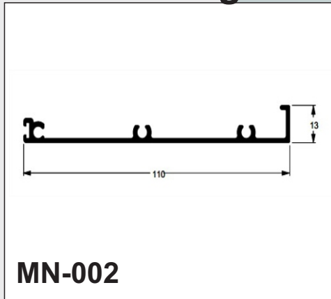
Inferior integrada
