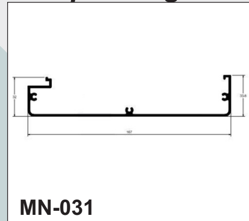
Tampa Integrada
