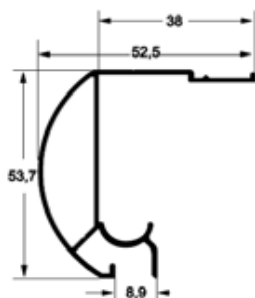
BX 200 - Trilho Superior Box
