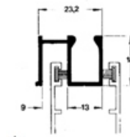
Z 074 - Perfil Z
