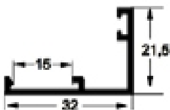
L 1026 - Baguetão
