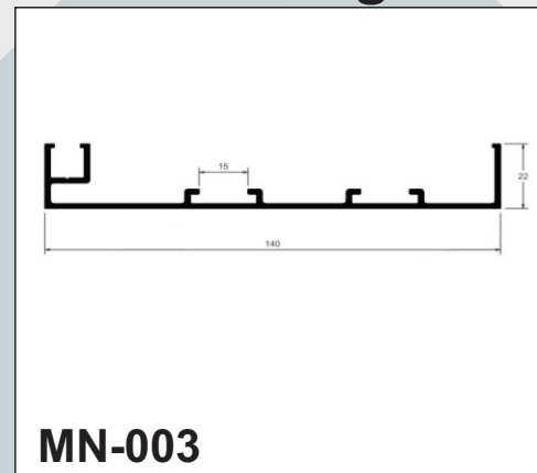
Lateral Integrada
